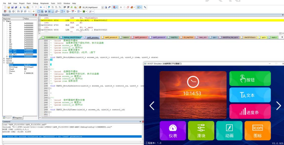
图 12-3 Keil 开发环境与虚拟串口屏绑定调试
