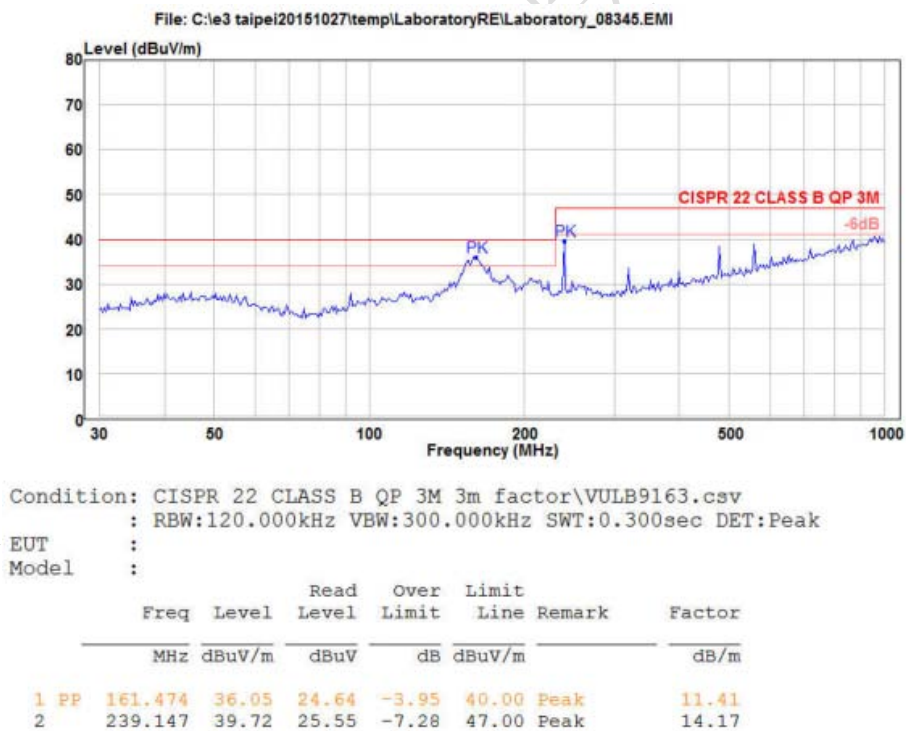
图 4-6 辐射测试水平方向
