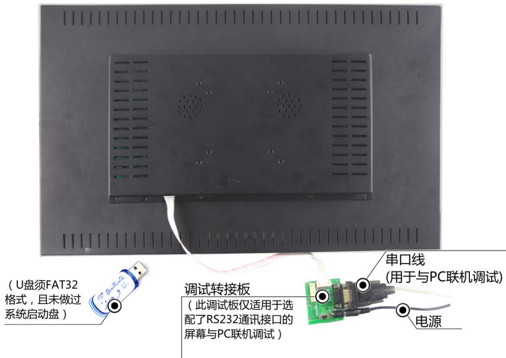
图 1-3 调试工具图
